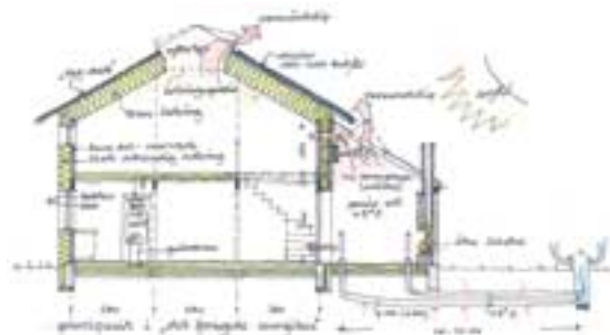
Skitsen viser det forslag til fremtidens parcelhus, som byggevirksomheden Forny et Energi har indsendt - www.fornyenergi.dk . Det er lykkedes at få dette hus klassificeret som lavenergihus kategori 1 efter bygningsreglementets nye beregningsmodeller - uden at sætte økologi og indeklima over styr.
